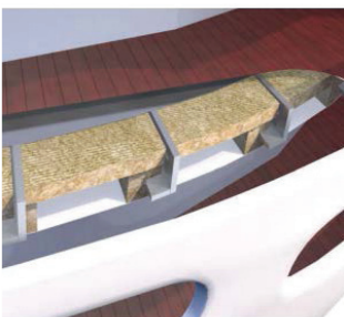
Esteras y tablones marinos Roxul SeaRox SL 600
